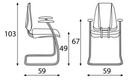
451/C Permanent contact mechanism. Meccanismo contatto permanente. 452/C 2 levers asynchro mech. Asincrono 2 leve. 453/C 3 levers asynchro mech. Asincrono 3 leve.
